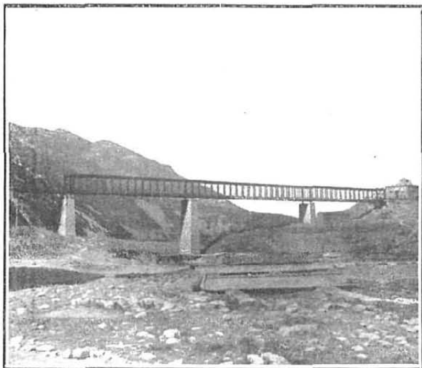
Puente de 180 metros de longitud que ha sido inaugurado hace pocos días en La Peña (Huesca) próximo a las obras del Pantano FOT. LARGINAGA
